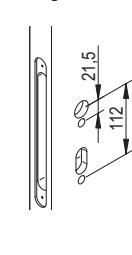
SH door configuration
