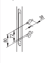
RO door configuration
