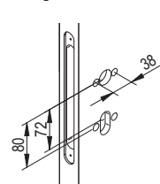
RO door configuration
