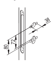
RO door configuration
