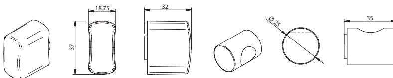
S thumbturn
